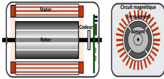
Fig. 2. PMSG scheme
